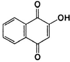
Lawsone
