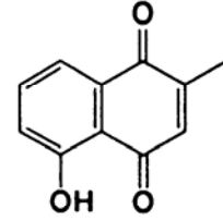
Plumbagin
