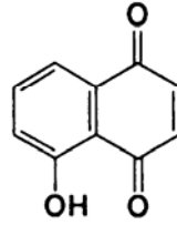
Juglone
