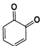
o -Quinone
