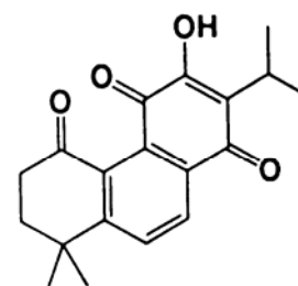
Miltionone (abietane-quinone)
