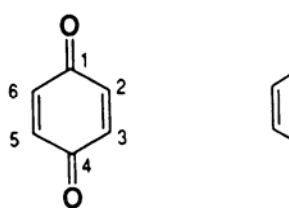
p -Quinone
